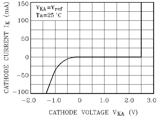
I_K - V_{KA}
