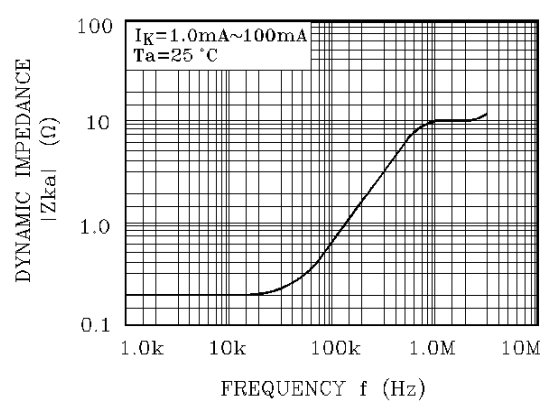
|Z_{ka}| - f
