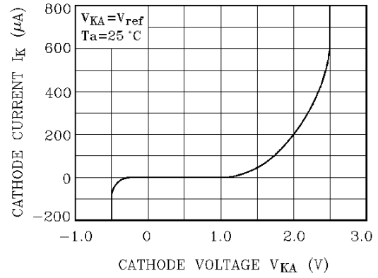
I_K - V_{KA}
