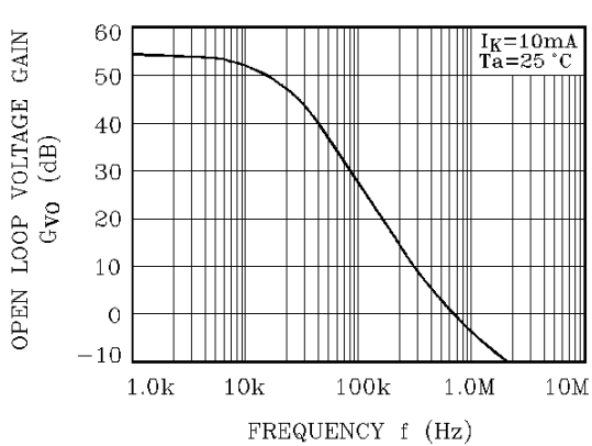
G_{v0} - f
